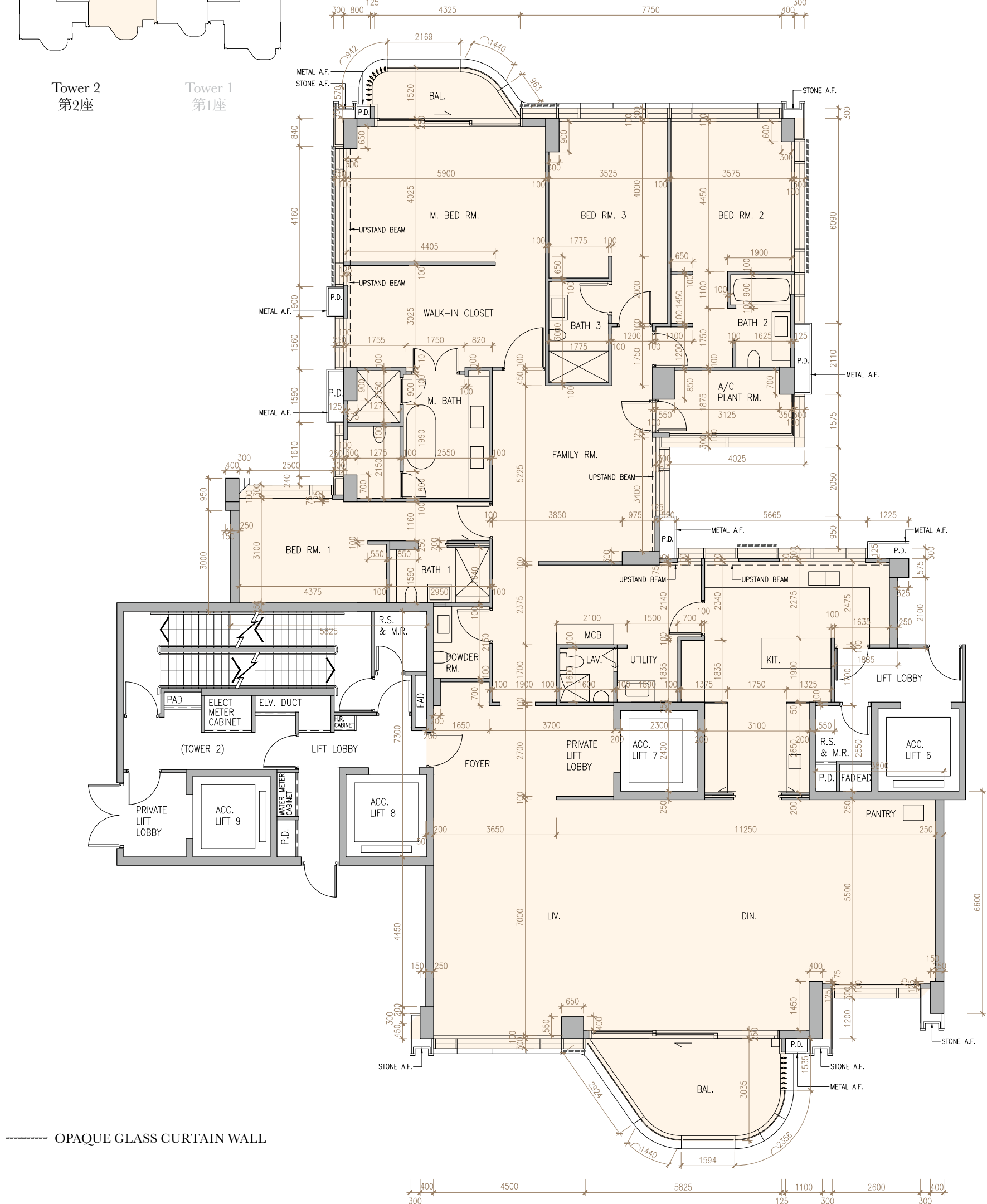
UNIT C 16/F FLOOR PLAN C 單位 16樓樓面平面圖
