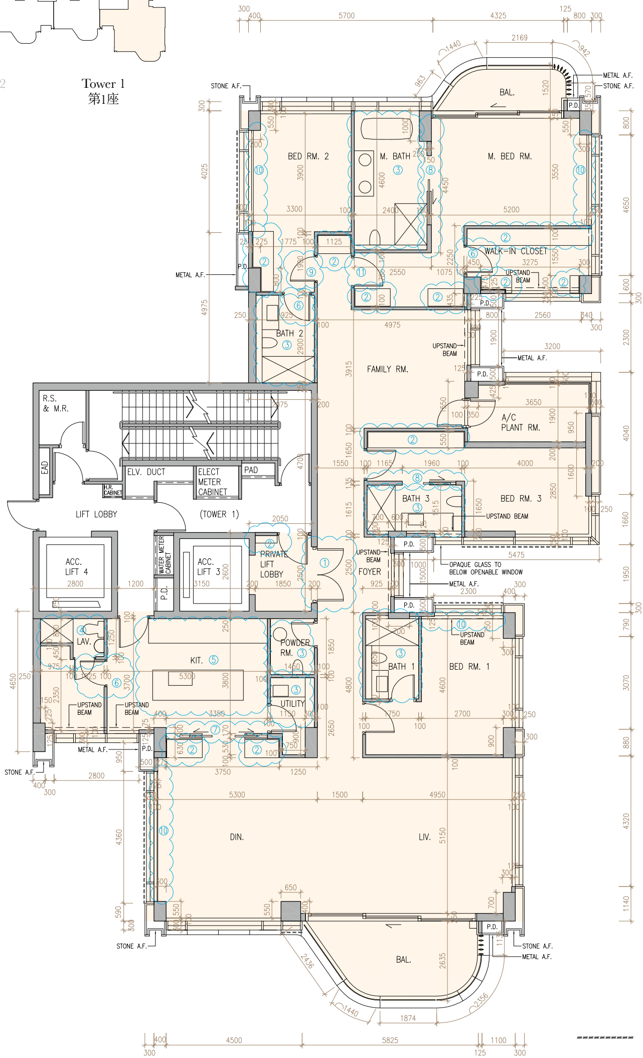
UNIT A 16/F FLOOR PLAN SHOWING LATEST LAYOUT A 單位 16樓現狀樓面平面圖
